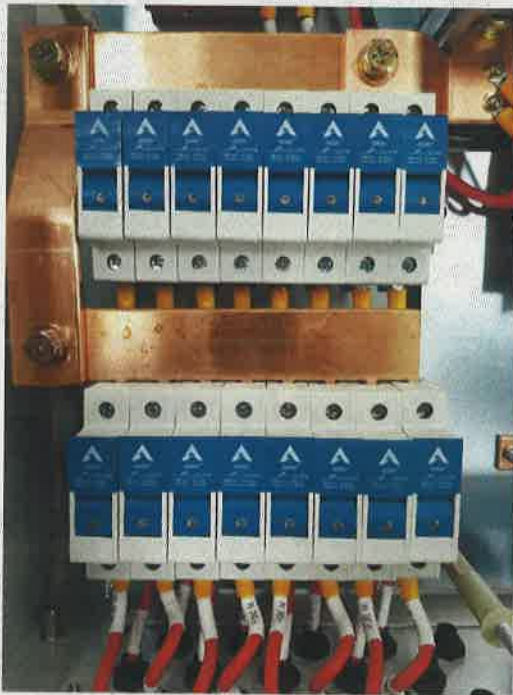
부품 - 퓨즈박스
