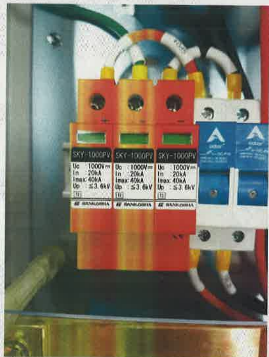
부품 - 서지보호기
