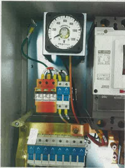
부품 - 내부배선
